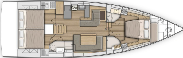
Versión 3 camarotes 3 cuartos de aseo:
