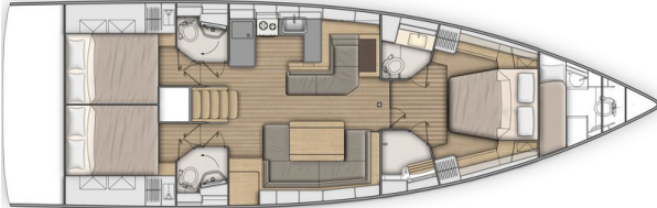
Versión 4 camarotes 2 cuartos de aseo:
