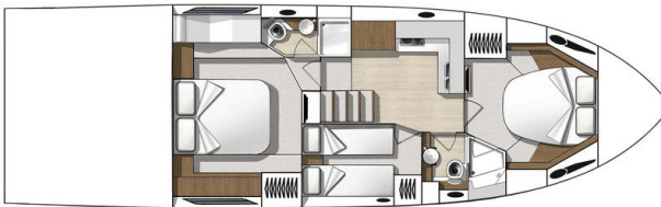
Versión 3 camarotes
