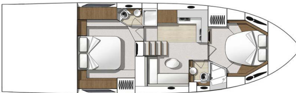
Versión 2 camarotes
