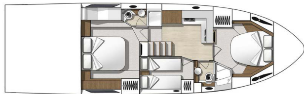
Versión 3 camarotes
